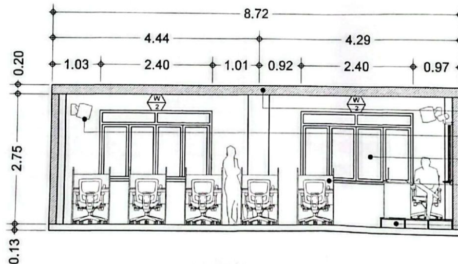
LONGITUDINAL SECTION SCALE 1 : 60 M.
