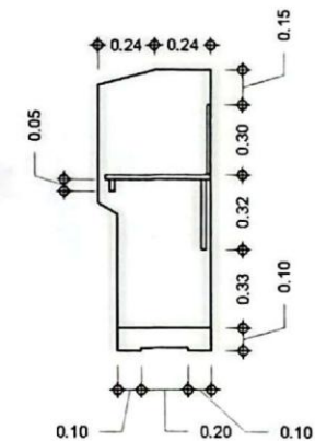
LONGITUDINAL SECTION
